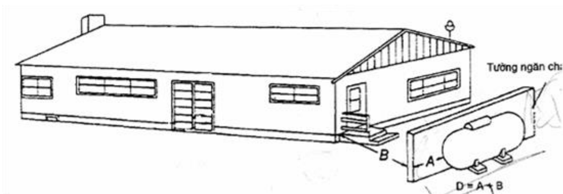
Hình 1 - Cách tính khoảng cách an toàn từ bồn chứa khí có tường ngăn cháy
