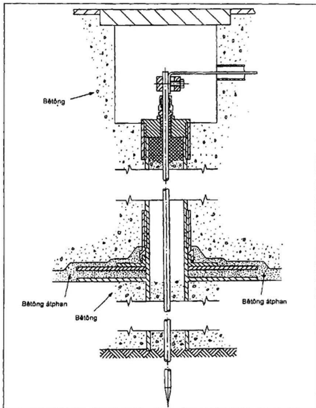
Hình 23 - Ví dụ về cọc nổi đất có lớp bọc được sử dụng trong kết cấu bê tông
