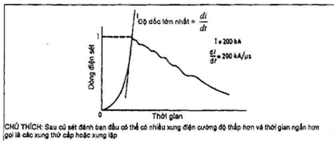
Hình C.15 - Đường đặc tính dòng sét âm
