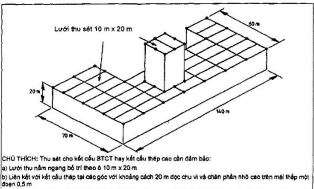
Hình 14 - Thu sét cho công trình có tháp cao dẫn điện
