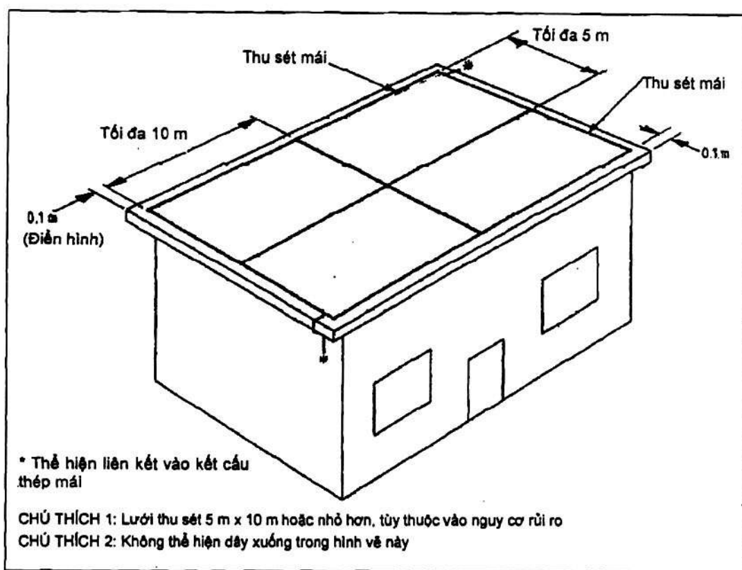
Hình 15 - Thu sét cho công trình có chứa các chất dễ gây cháy nổ
