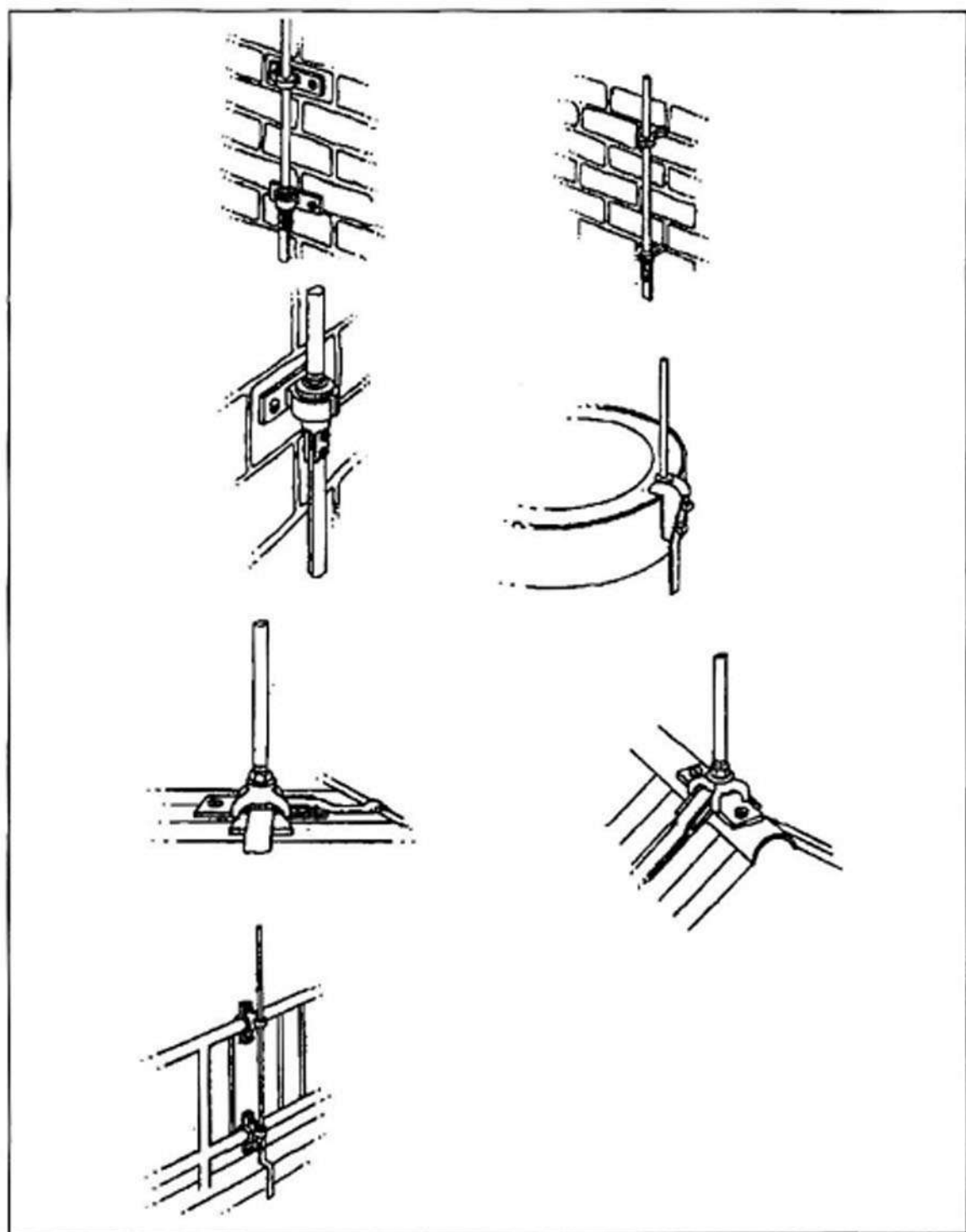
Hình 8 - Các kiểu kìm thu sét điện hình
