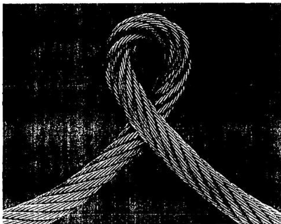
Hình B.17 - Cáp bị xoắn vặn
