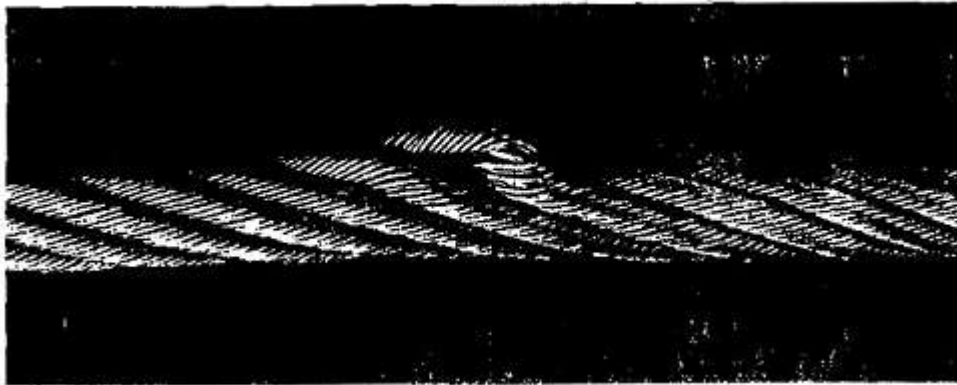
Hình B.4 - Tào cáp nhô ra hoặc bị bóp méo
