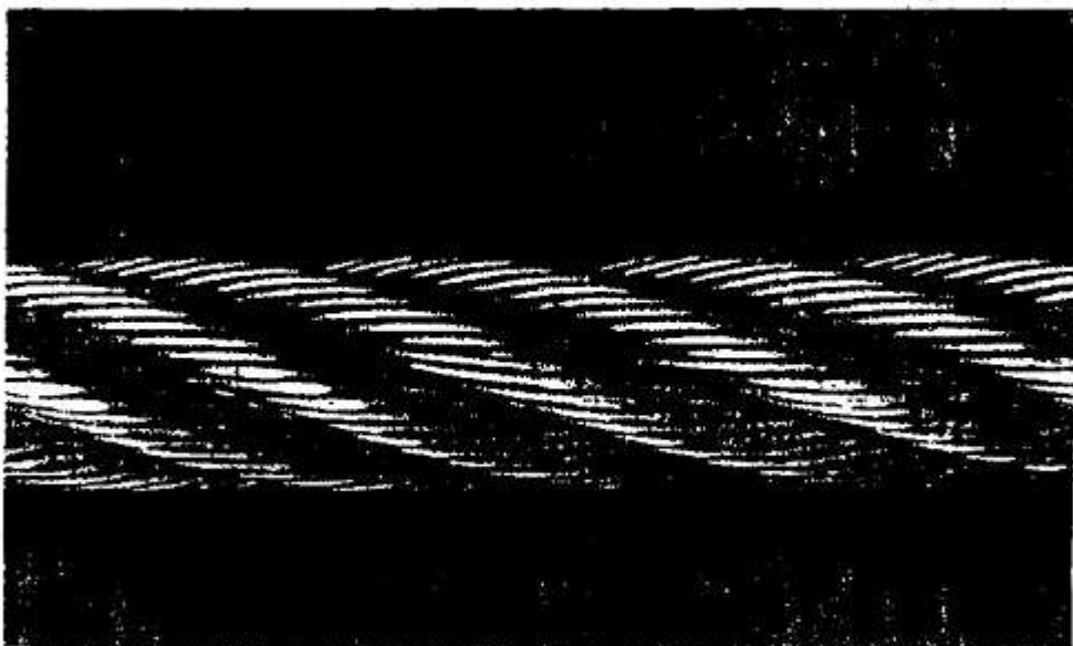
Hình B.14 - Đứt sợi vùng lõi
