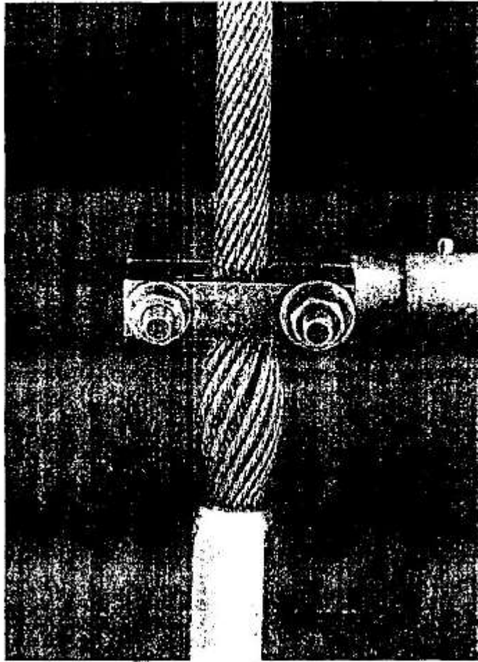
b) Ở đoạn ngay sát vị trí cố định đầu cáp (không bị lực căng)
