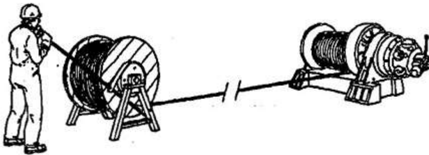
Hình 4 - Ví dụ về chuyển cáp từ phía dưới tang cáp đến phía dưới tang (của cần trực) có kiểm soát lực căng
