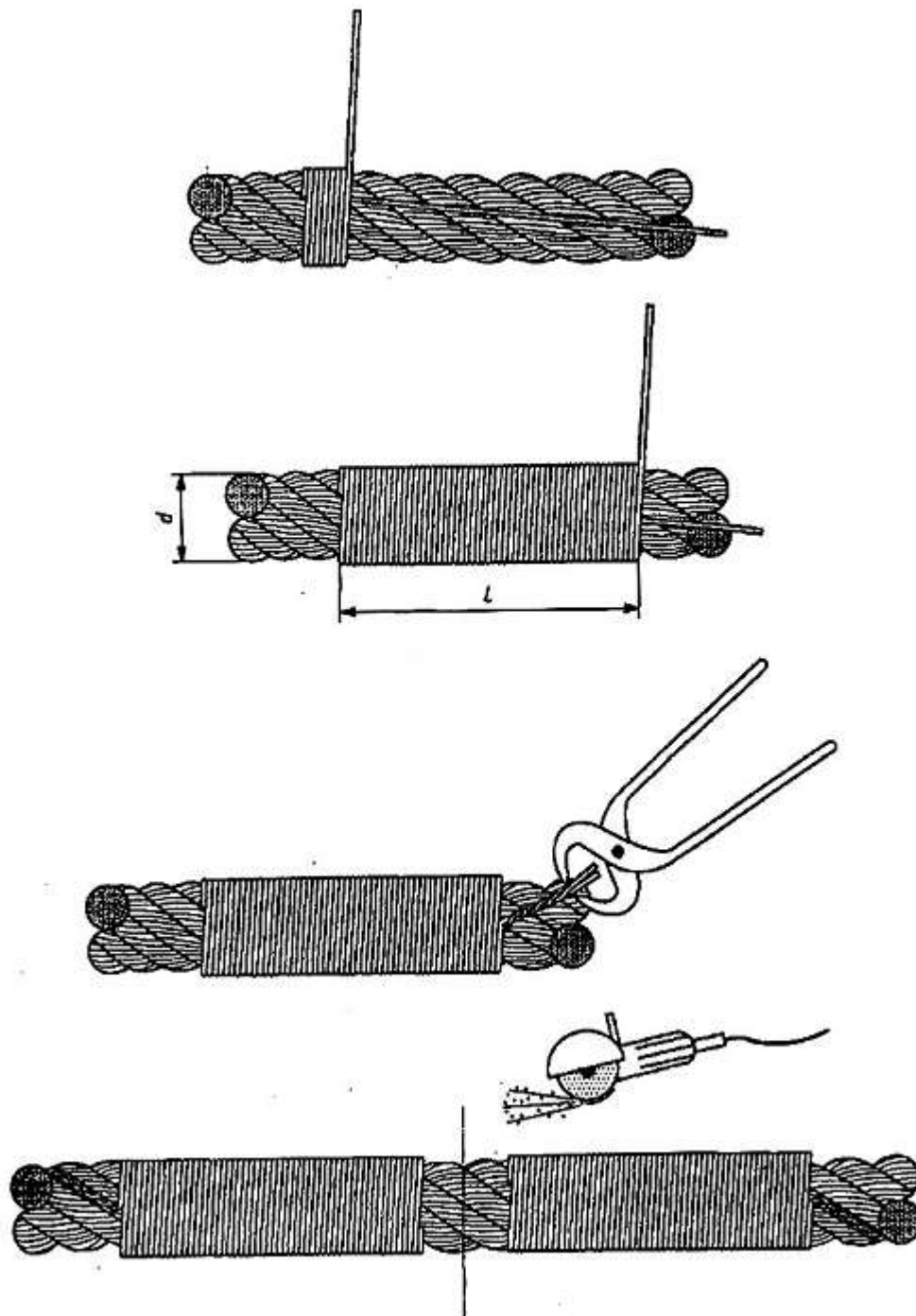
Hình 1 - Chống xoắn cáp trước khi cắt đối với cáp một lớp
