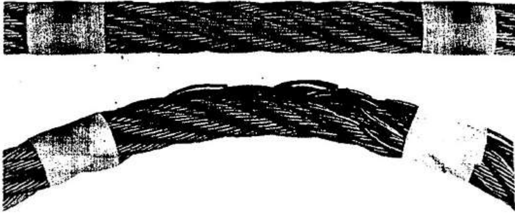
Hình 7 - Uốn cong cáp thường làm lộ sợi đứt ẩn tại vùng khe giữa các tào cáp
